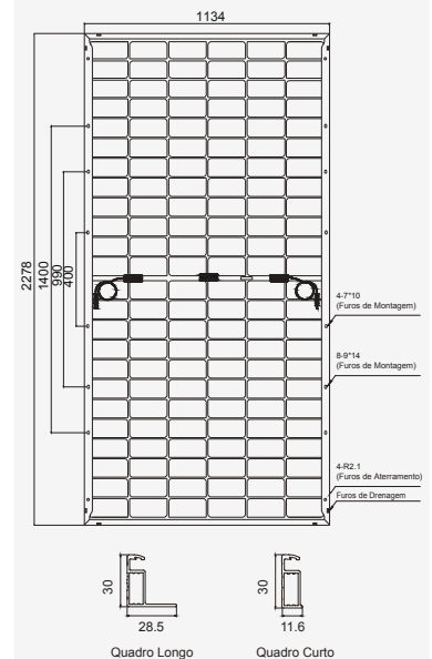
Vista Traseira
